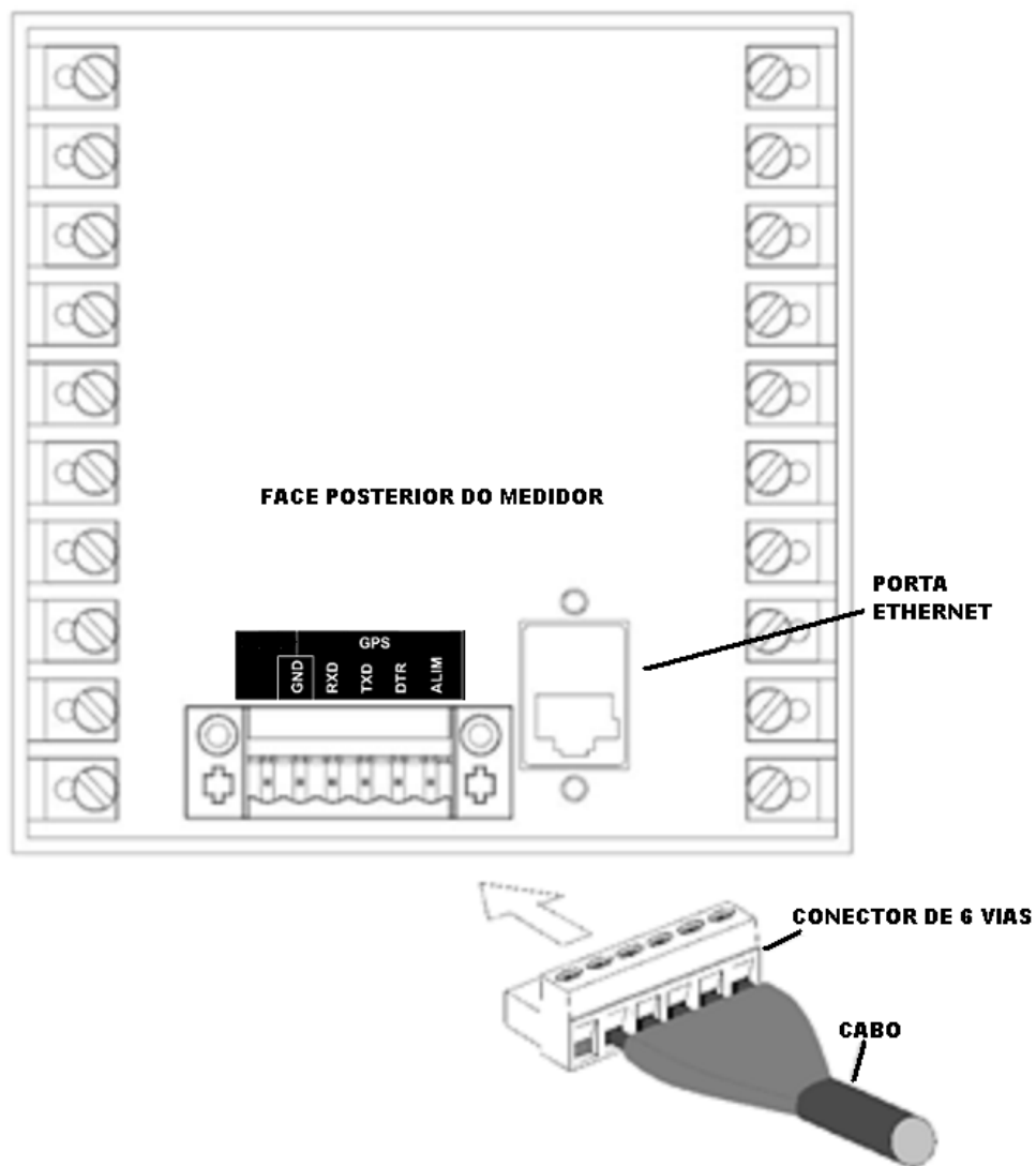
Figura 3.7 - Conexão do cabo aos medidores ELO2183 de embutir
