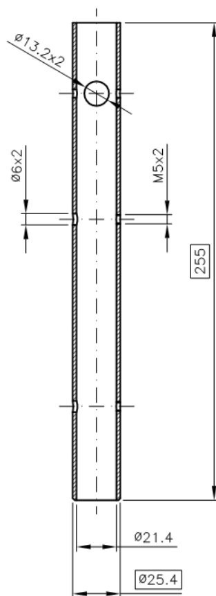
Figura 3.2 – Diagrama de fixação do ELO588
