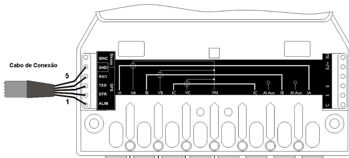
Figura 3.5 - Conexão do cabo aos medidores ELO2180 de sobrepor
