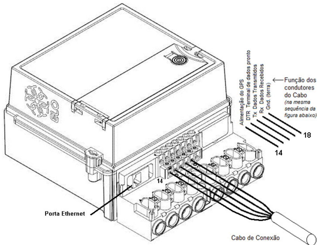
Figura 3.8 - Conexão do cabo aos medidores de sobrepor
