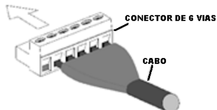
Figura 3.6 - Conexão do cabo aos medidores ELO2180 de embutir
