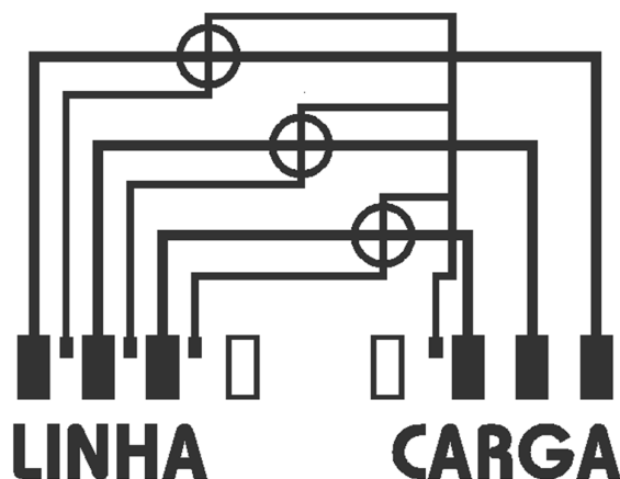
Figura 3.2 – Esquema de Ligação do ELO2133TI
