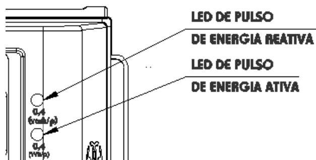
Figura 4.1 – Localização dos LEDs de calibração de energia ativa e reativa.
