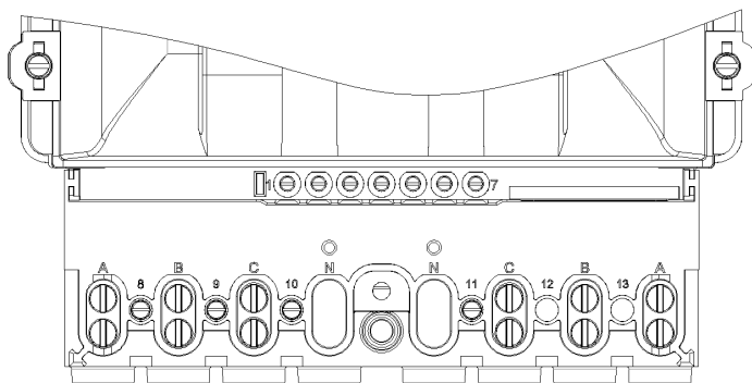
Figura 2.4 - Terminais do ELO2133TI
