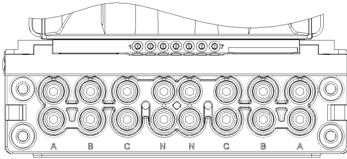
Figura 2.4 - Terminais do ELO2133T200.
