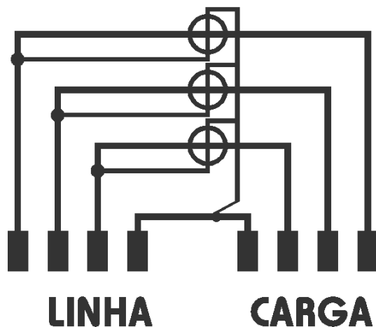
Figura 3.2 – Esquema de Ligação do ELO2133T200.
