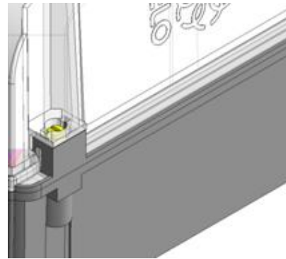
Figura 2.3 – Detalhe do ponto de lacre de fabricação e/ou verificação metrológica.
