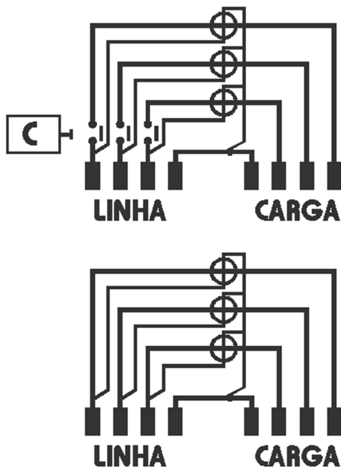
Figura 3.2 – Esquema de Ligação do ELO2133T com e sem relé de gestão de cargas
