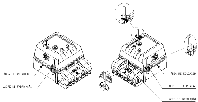
Figura 2.2 - Demonstrativo dos Lacres do ELO2133T.
