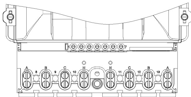
Figura 2.4 - Terminais do ELO2133T
