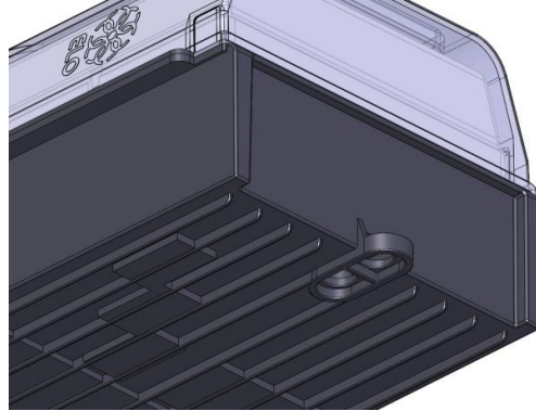
Figura 3.1 – Furo embutido na base do medidor ELO2132T
