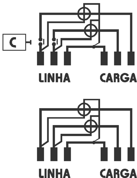
Figura 3.2 – Esquema de Ligação do ELO2132T com e sem relé de gestão de cargas
