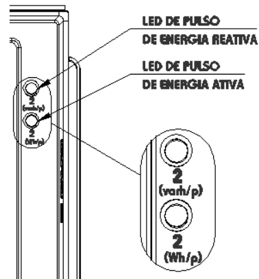
Figura 4.1 – Localização dos LEDs de calibração de energia ativa e reativa.
