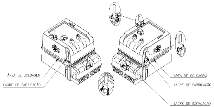
Figura 2.2 - Demonstrativo dos Lacres do ELO2132T.
