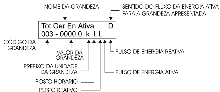
Figura 5.1 – Mostrador no modo Normal do ELO2127.
