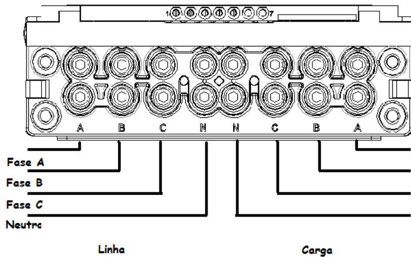
Figura 3.2 - Ligações no bloco de terminais
