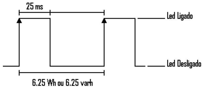
Figura 7.2 - Forma de onda dos pulsos de calibração.
