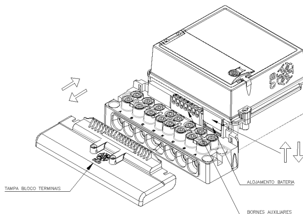
Figura 3.1 – Detalhe da tampa do bloco de terminais do ELO2127.
