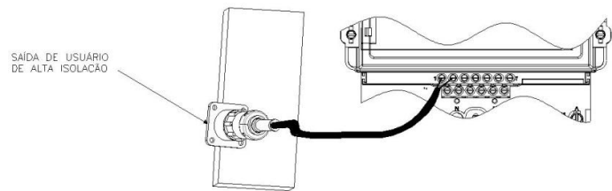
Figura 3.11 – Conexão da saída de usuário do ELO2127 através de um cabo de alta isolamento (óptico).
