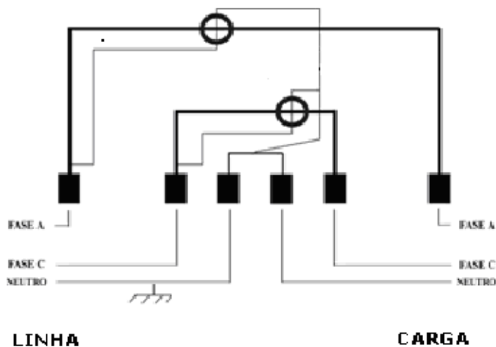
Figura 3.2 – Esquema de ligação do ELO2102L.
