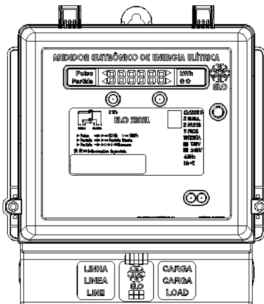
Figura 2.3 - Vista frontal do ELO2102L.
