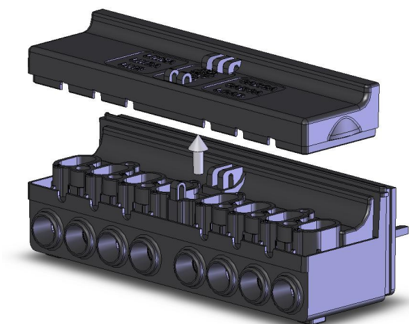
Figura 2.7 – Detalhe do bloco de terminais do ELO2102L
