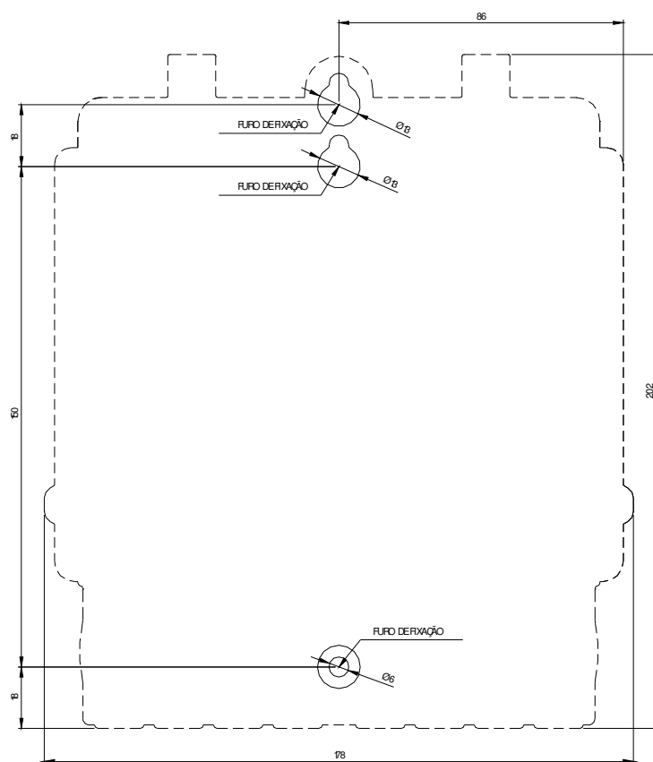
Figura 3.1- Pontos de fixação do ELO2102L.
