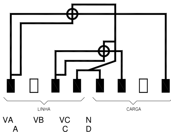
Figura 2.8 – Esquema dos terminais do ELO2102L
