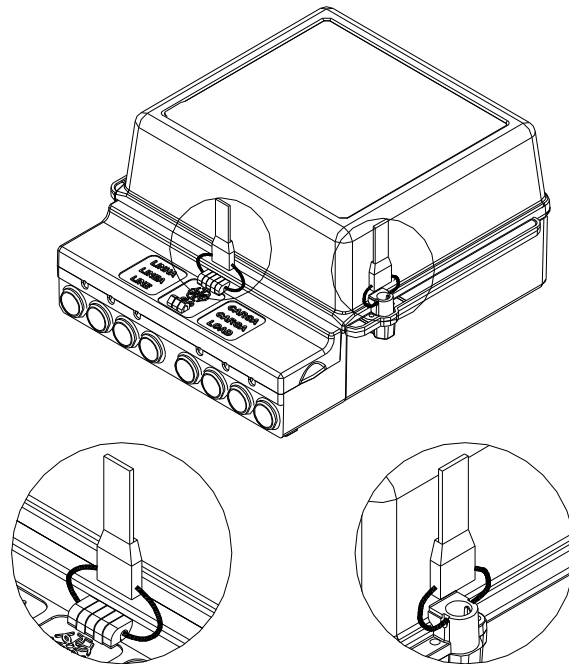
Figura 2.5 - Detalhe dos Lacs do ELO2102L.
