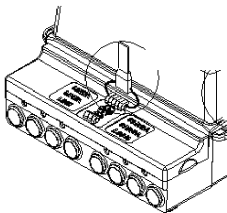
Figura 2.6 – Acesso ao bloco de terminais do ELO2102L
