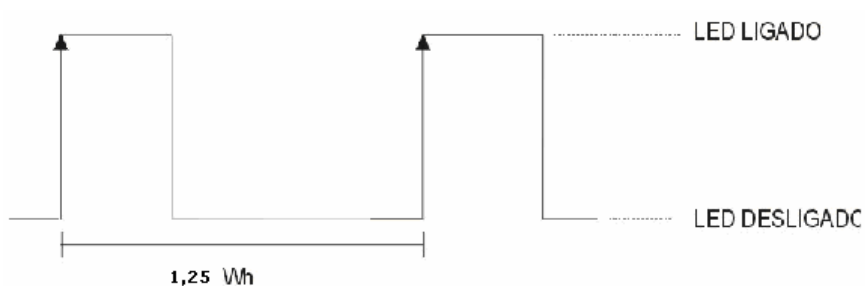
Figura 4.1 - Forma de onda dos pulsos de calibração.
