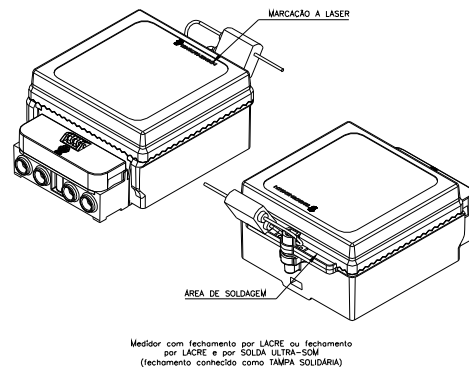
Figura 2.2 - Demonstrativo do Lacre do ELO2101A.
