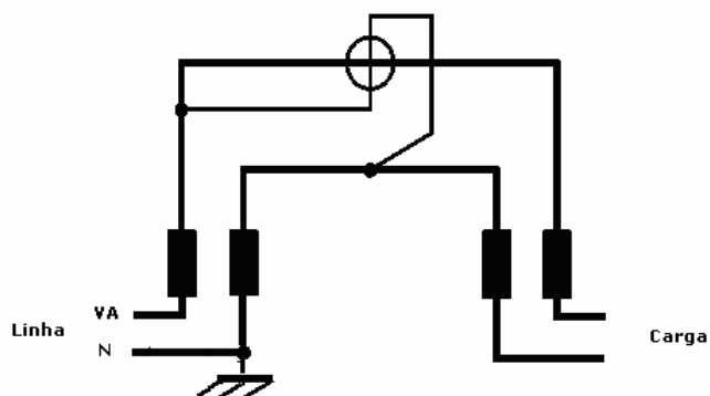
Figura 3.2 – Esquema de ligação do ELO2101A.
