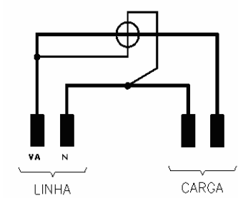
Figura 2.4 - Terminais do ELO2101A
